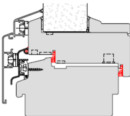
Alu-Vorsatzschalen/ Holz-Alu-Konstruktionen (Dichtungsebenen und Profilabmessungen des Brandschutzelements dürfen nicht beeinträchtigt sein)
