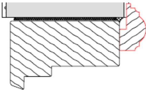
Verleistung/ Profile zum Fensterrahmen bzw. Abdecken der Bauanschlussfuge
