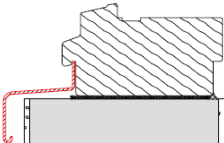
Fensterbänke/ Fensterbleche zum Fensterrahmen
